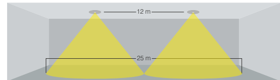
Višestruka instalacija: Izlazni put osvijetljen sa 1 lux - H 3m Multiple installation: Exit path illuminated with 1 lux - H 3m
