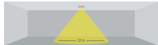
Jedan modul: Izlazni put osvijetljen sa 1 lux - H 3m Single unit: Exit path illuminated with 1 lux - H 3m
